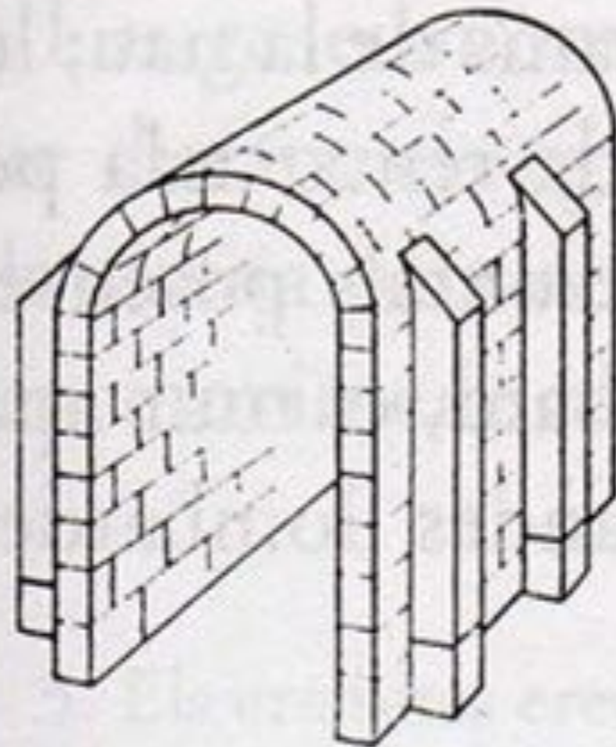
Volta de canó amb contraforts extersors
