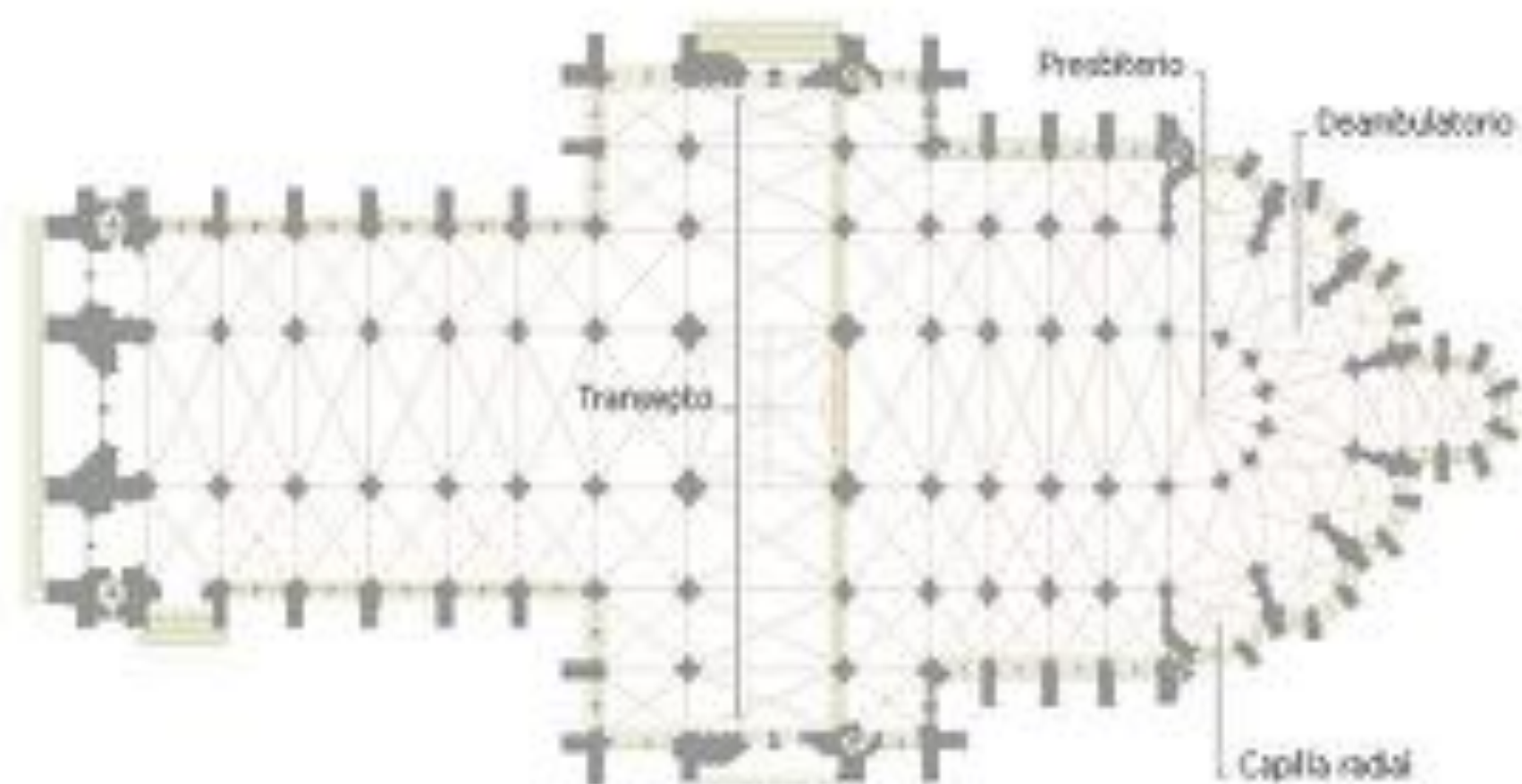
Planta de la catedral de Amiens
